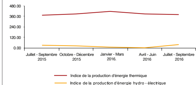
Indice de la production d'énergie thermique et hydro électrique (1986 - 87=100)
